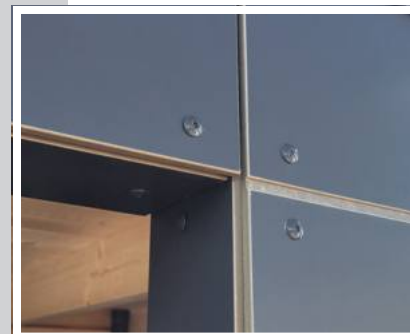
Wetterfeste Fassade aus HPL und Dachkantenprofil aus Aluminium.
